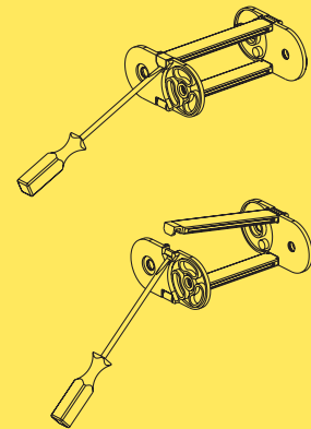
Rahmensteg montieren
