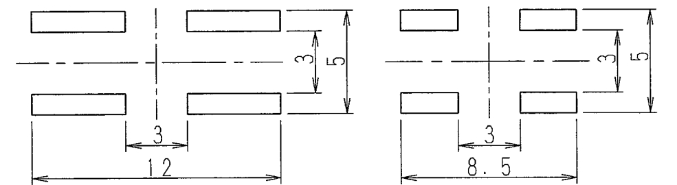
a) DIMENSION FOR FLOW SOLDERING フロー溶着パターン図 b) DIMENSION FOR REFLOW SOLDERING リフロー溶着パターン図
