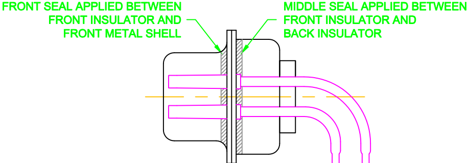
DETAIL A-A
