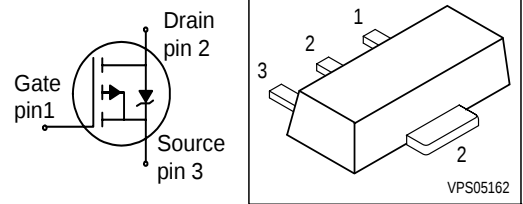
SOT89
