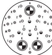
24-20 10#20 13#16 4#12 3 TWINAX #8 (N)
