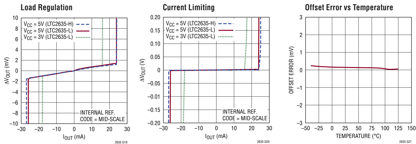
LTC2635
