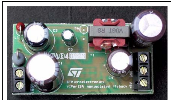
STEVAL-ISA006V1
