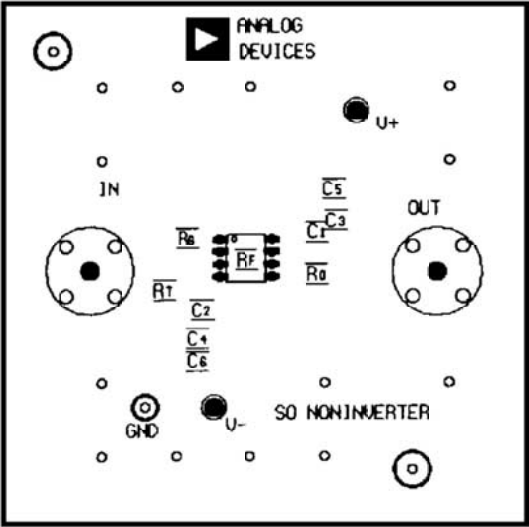
SOIC (R) NONINVERTER
