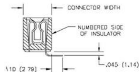
CONTACT CODE 553
