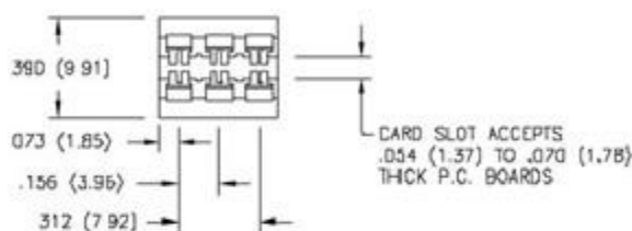
6 CONTACT CENTRE MODULE
