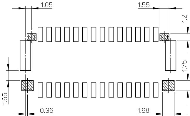
△8 パターン禁止エリア (参考) PATTERN PROHIBITION AREA (REF.)
