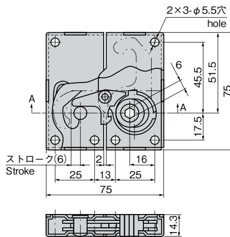
A-A 断面 Cross section
