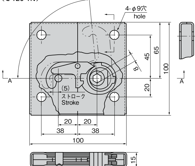
A-A 断面 Cross section
