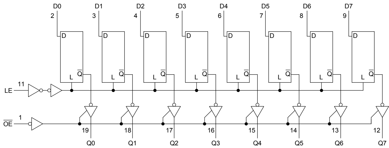
システム図
