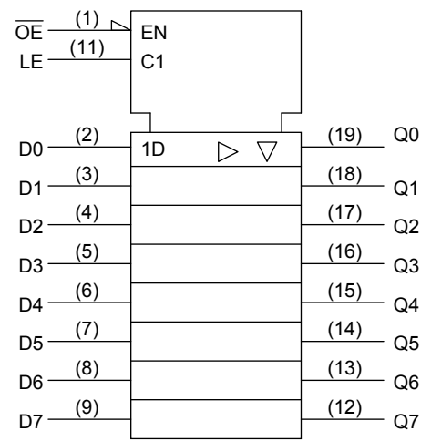
論理図
