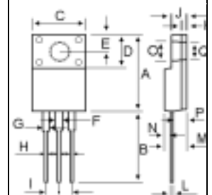
ITO-220
