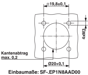
Einbaumaße: SF-EP1N8AAD00
