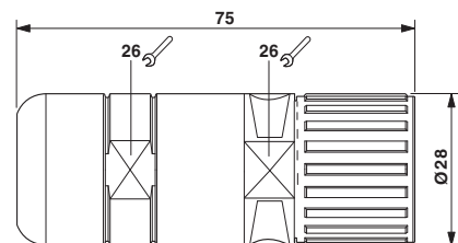
SF-.ES1N8A8L..
