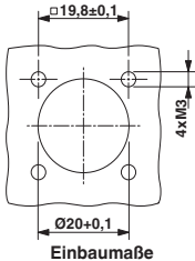
Einbaumaße
