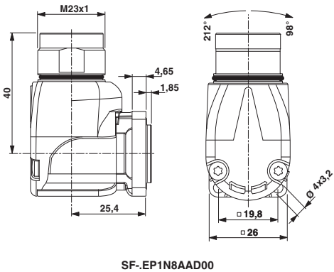
SF-EP1N8AAD00
