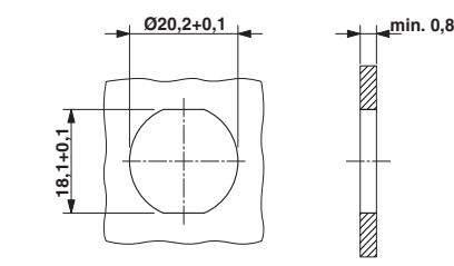
Einbaumaße: ST-17.1N8AH100S, Bohrung mit Verdrehenschutz und Kontermutter (Empfehlung bei Einbau in Stahlblechwand)
