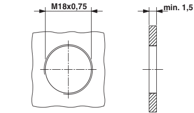
Einbaumaße: ST-17.1N8A6100S, Durchgangsbohrung mit Gewinde (Empfehlung bei Einbau in Stahlblechwand)
