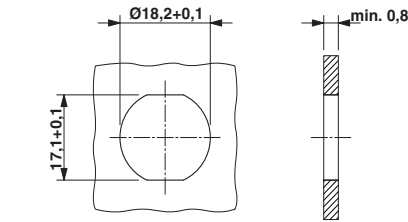
Einbaumaße: ST-17.1N8A6100S, Bohrung mit Verdrehenschutz und Kontermutter (Empfehlung bei Einbau in Stahlblechwand)
