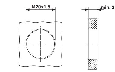
Einbaumaße: ST-17.1N8AH100S, Durchgangsbohrung mit Gewinde (Empfehlung bei Einbau in Stahlblechwand)
