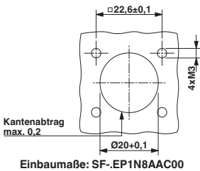
Einbaumaße: SF-EP1N8AAC00
