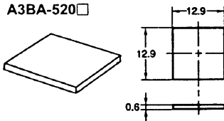
A3BA-520□
