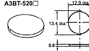
A3BT-520□
