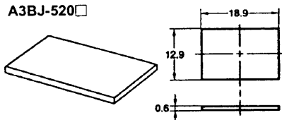
A3BJ-520□
