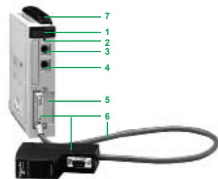
TSX P57 0244M
