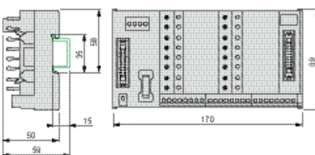
ABE 7TES160
