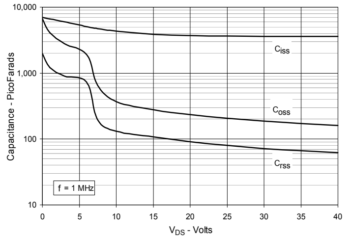
Fig. 14. Capacitance
