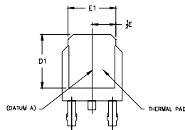
VIEW A-A
