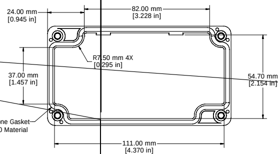
LID - INSIDE
