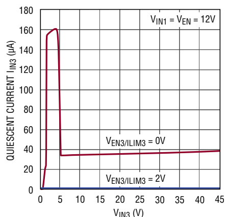
LDOs: 5V Quiescent Current IN3
