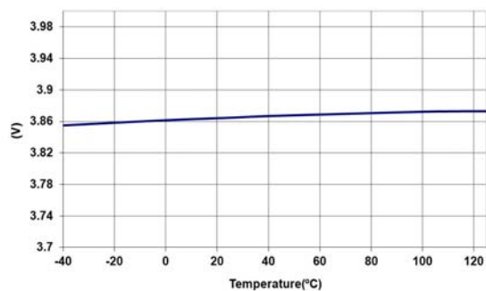
Vcc_UVLO_Stop
