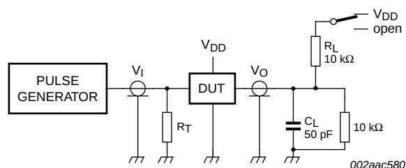
Fig 15. Test circuitry for enable/disable times, SDOUT ( t_{en}(SDOUT) and t_{dis}(SDOUT) )
