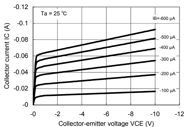
IC - VCE
