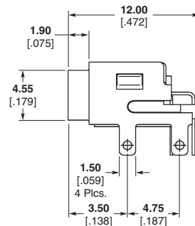
Sec. A-A
