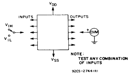
Fig. 14 - Input voltage.
