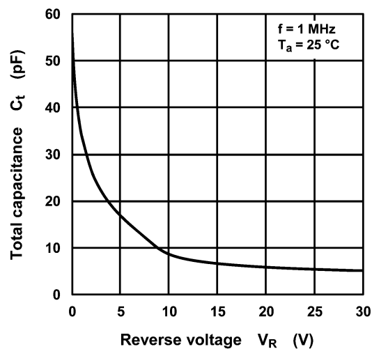
Fig. 8.3 C_t - V_R
