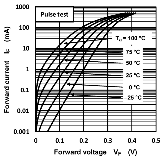
Fig. 8.1 I_F - V_F
