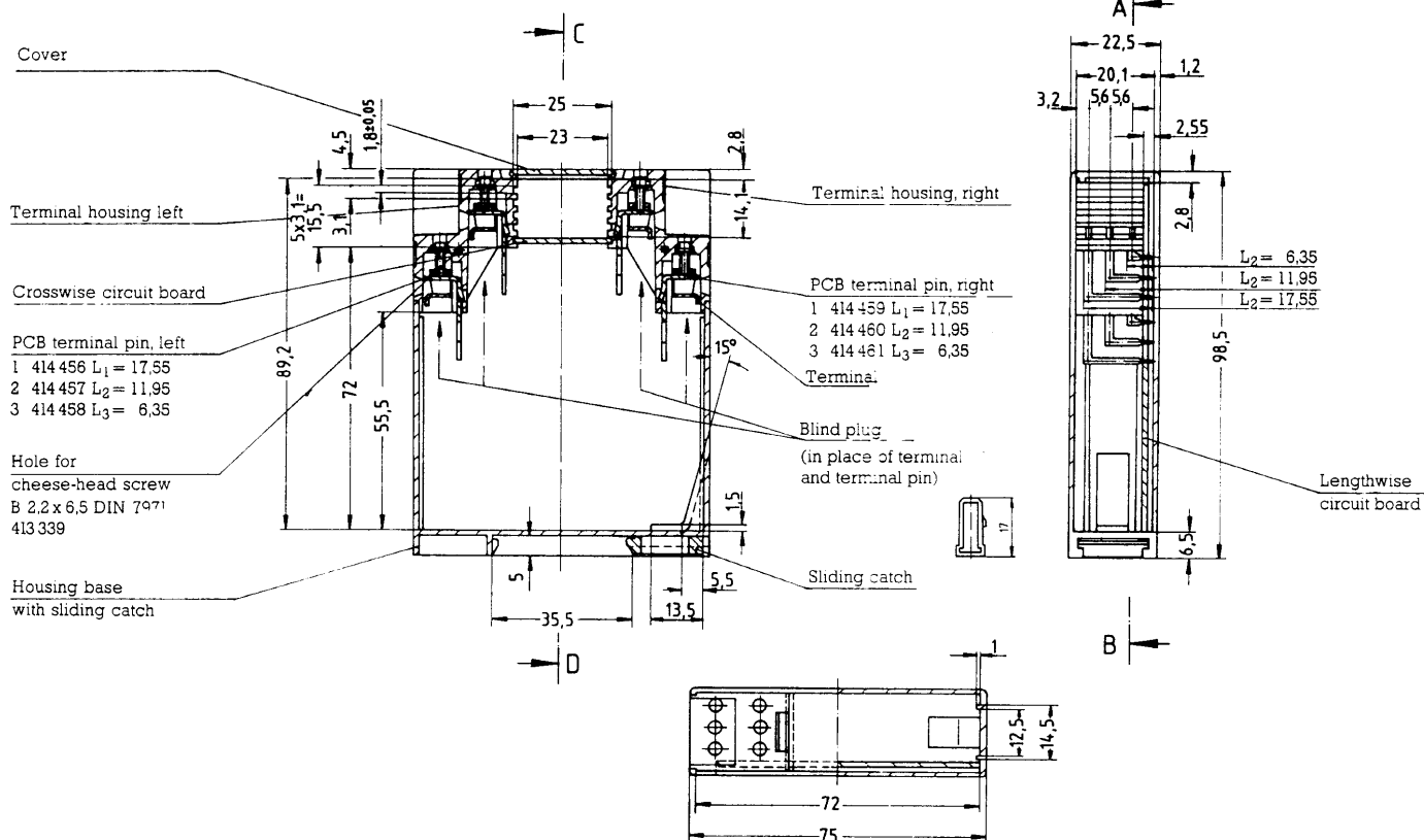
Section C-D
