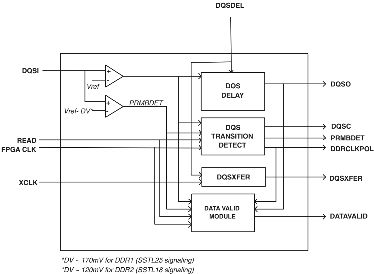
Figure 12-8. DQSBUFC Function
