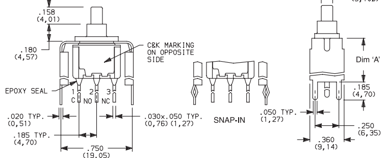
8121SD3_GE SPDT
