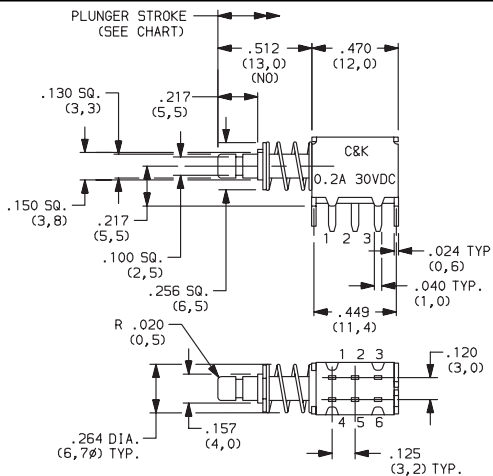
PN21LASA03QE DPDT
