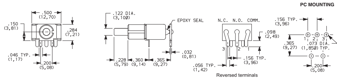
8121SD9R2GE SPDT
