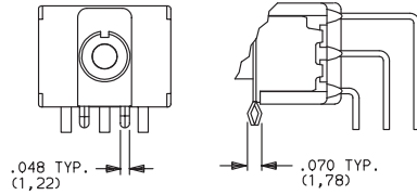
8321SD9AV2GE 3PDT
