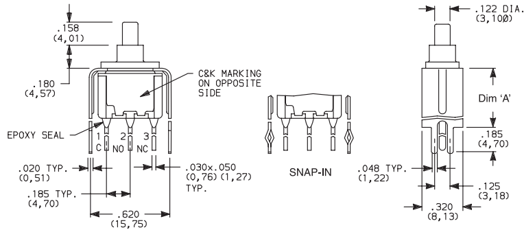
8121SD3_GE SPDT
