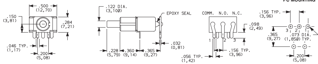
8121SD9RGE SPDT
