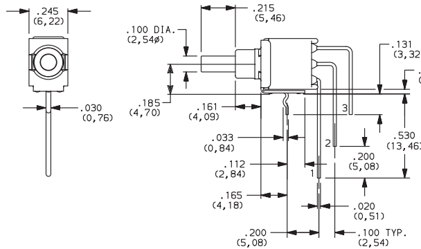
EP12SD1AV3BE SPST
