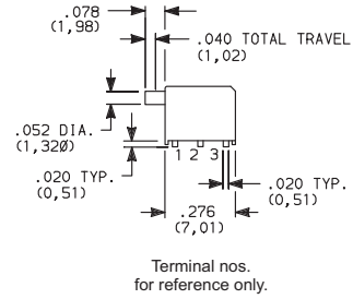
GP12MSCBE SPDT
