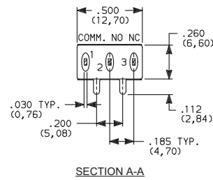
E121SD1AGE SPDT
