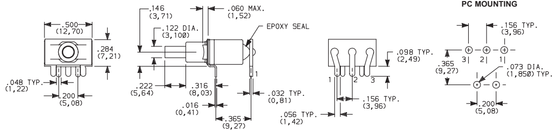
E112SD1R2BE SPDT
