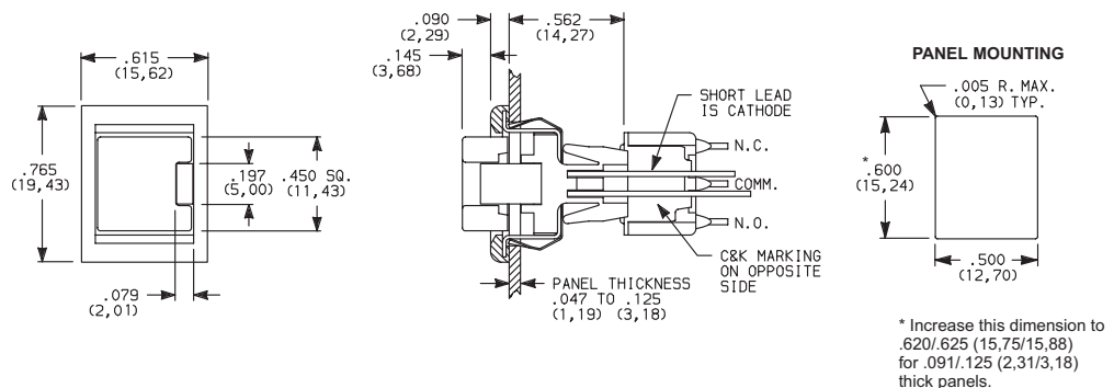
8161J86ZQE223 SPDT
