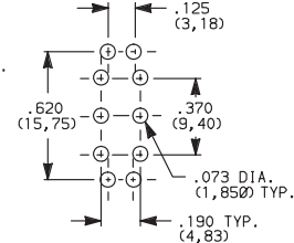
E221SD3_GE DPDT
