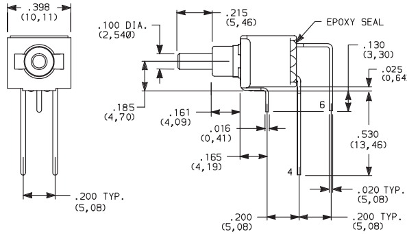
EP21SD1AVBE DPST
