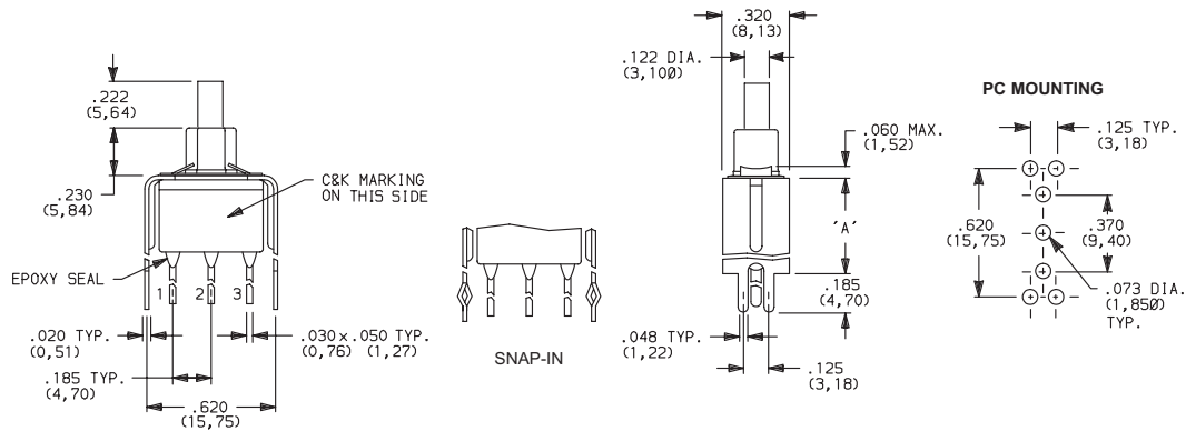
E112SD1_BE SPDT
