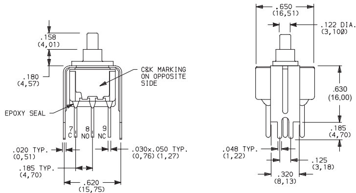
8321SD3V4GE 3PDT
