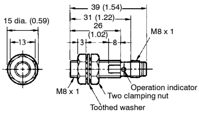
Fig. 20: E2E-X1R5E□-M3/F□-M3-N
