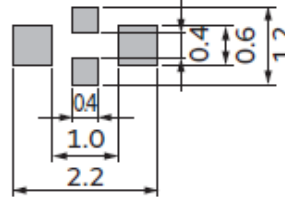
NFM18CC/18PC
