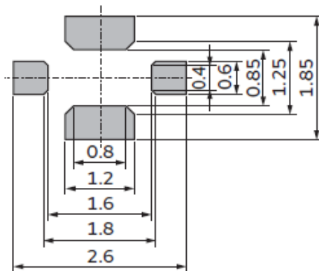
NFM31PC/31KC
