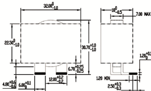
PQ3218-3R3-70-T | 3.3 \mu H
