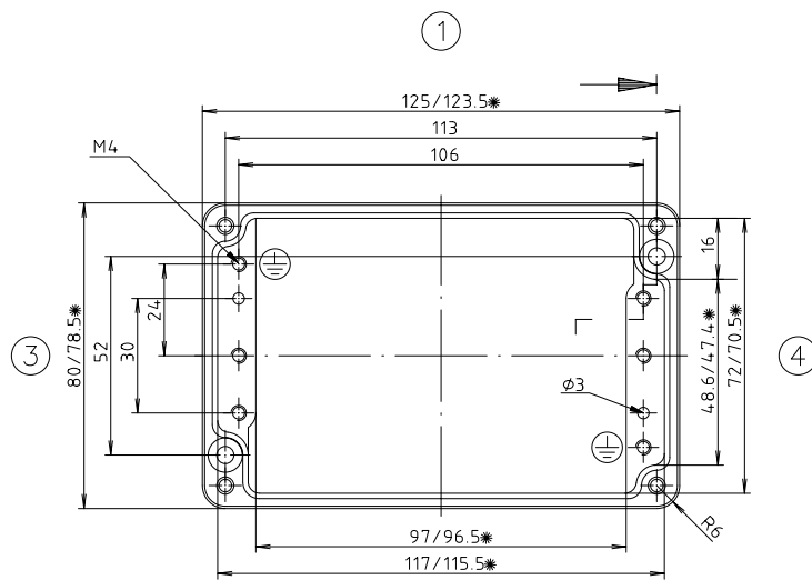
Unterteil
