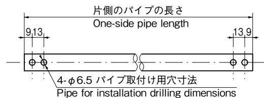
パイプ取付け用穴寸法 Pipe for installation drilling dimensions
