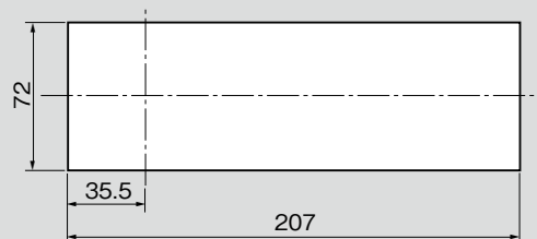
パネル穴明け寸法 Panel drilling dimensions
