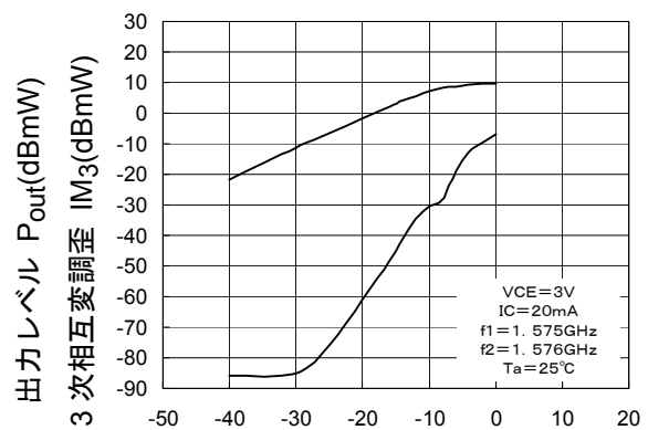
P_{\text{out}}, \text{IM}_3\text{-}P_{\text{in}}
