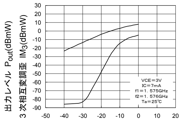
P_{\text{out}}, \text{IM}_3\text{-}P_{\text{in}}
