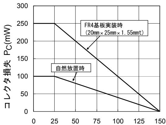
P_C - T_a
