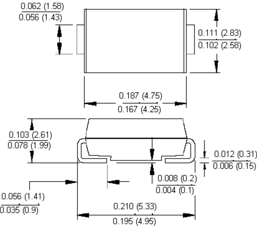
Dimensions : Inches (Millimetres)
