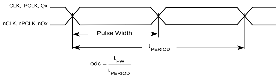
FIGURE 8 - odc & t_{PERIOD}
