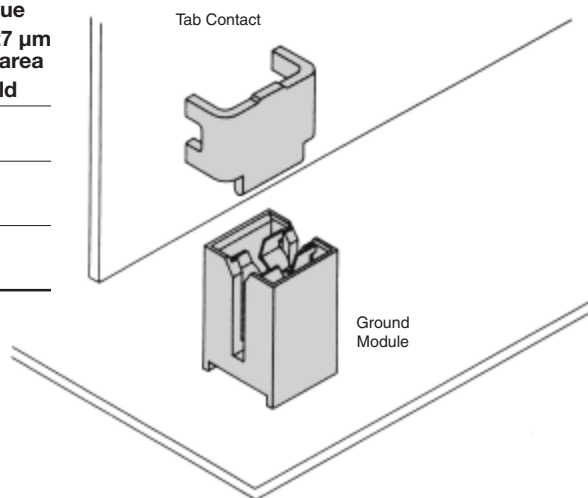
Tab Contact
