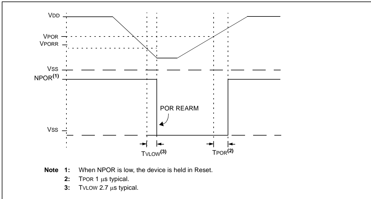
FIGURE 27-1: POR AND POR REARM WITH SLOW RISING V_{DD}
