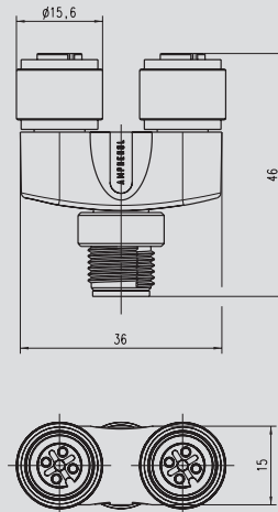
Y-Distributor 1x pin / 2x sockets
