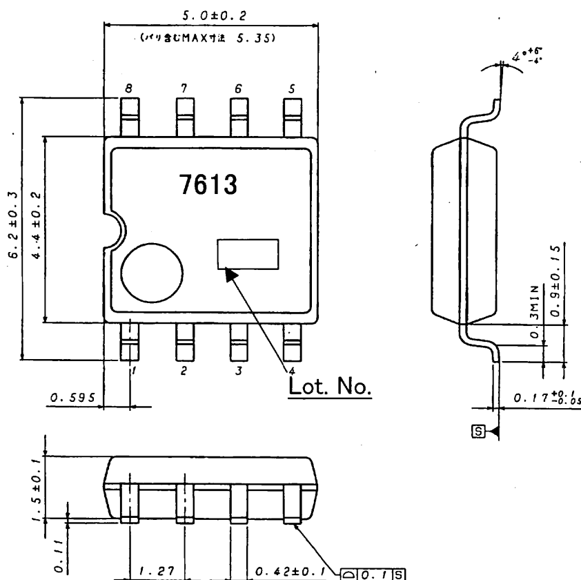
SOP8 (Unit:mm)
