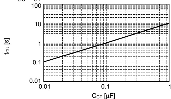
11. t_{CU}-C_{CT}
