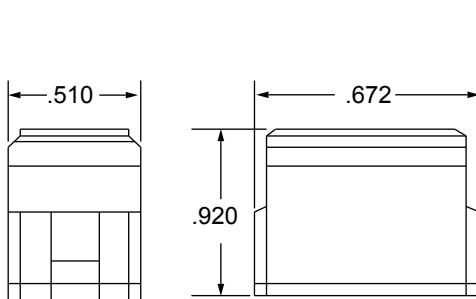
CTD16 Module
