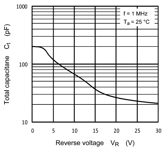
Fig. 9.3 C_t - V_R
