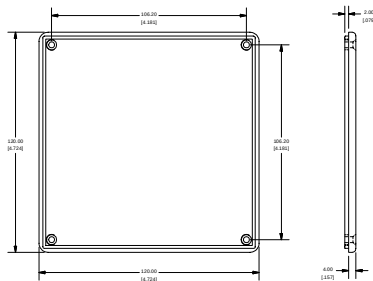
BOTTOM OF LID
