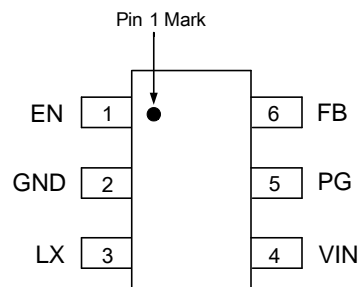
TSOT26
