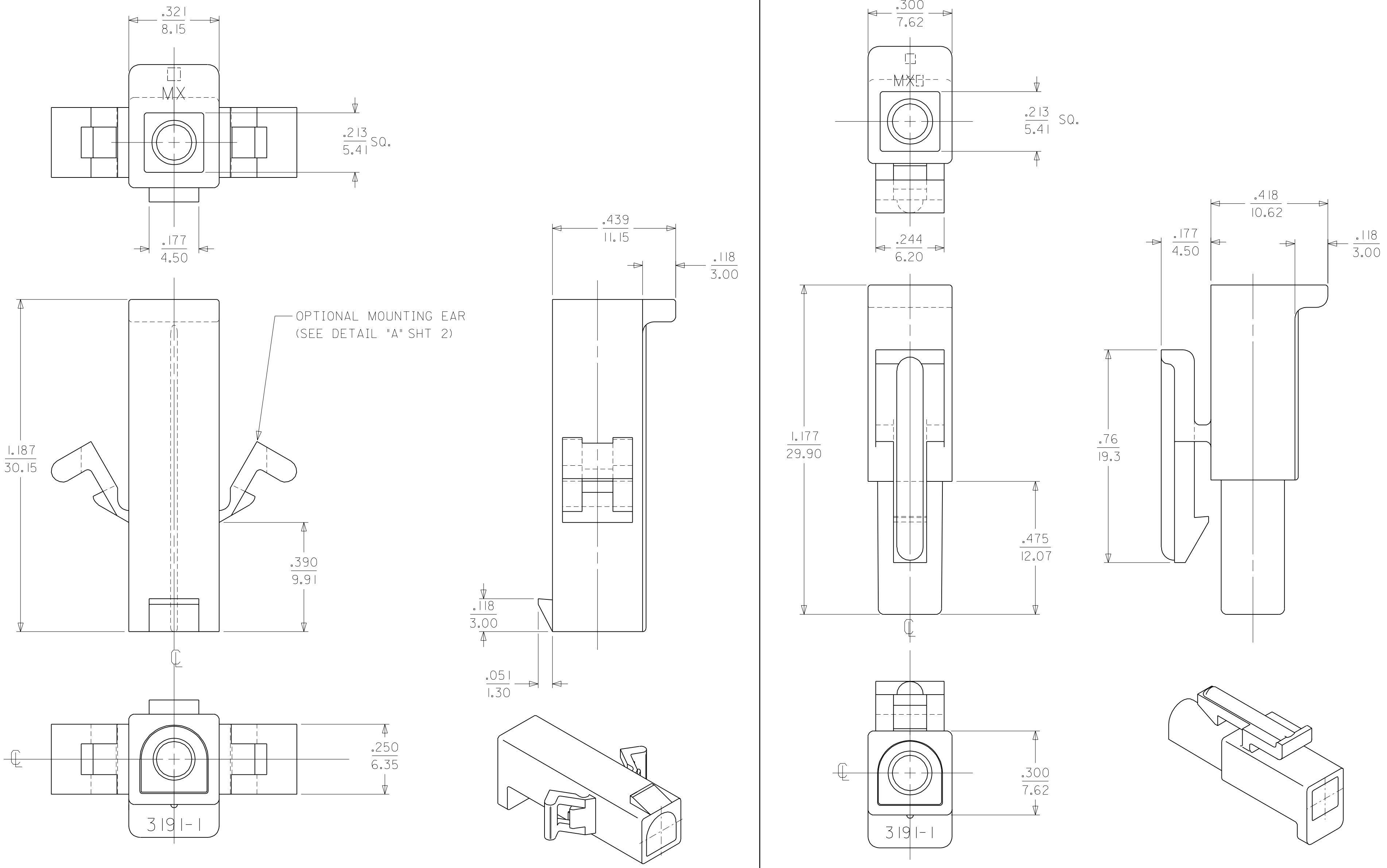
RECEPTACLE
