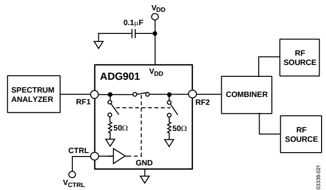
Figure 21. IP_3
