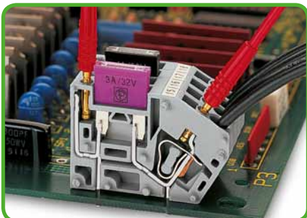
Prüfen - Sicherungsklemme
