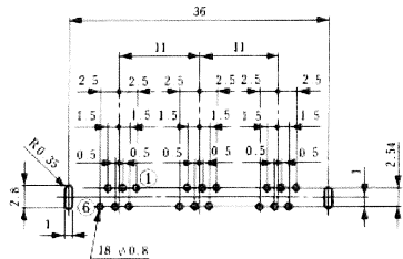
TM2REA-1818 (50)
