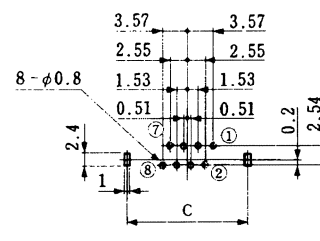
TM5RJ3-88(50)
