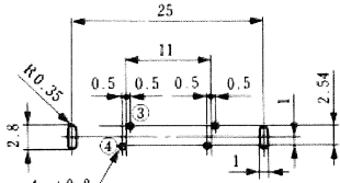
TM2REA-1204 (50)
